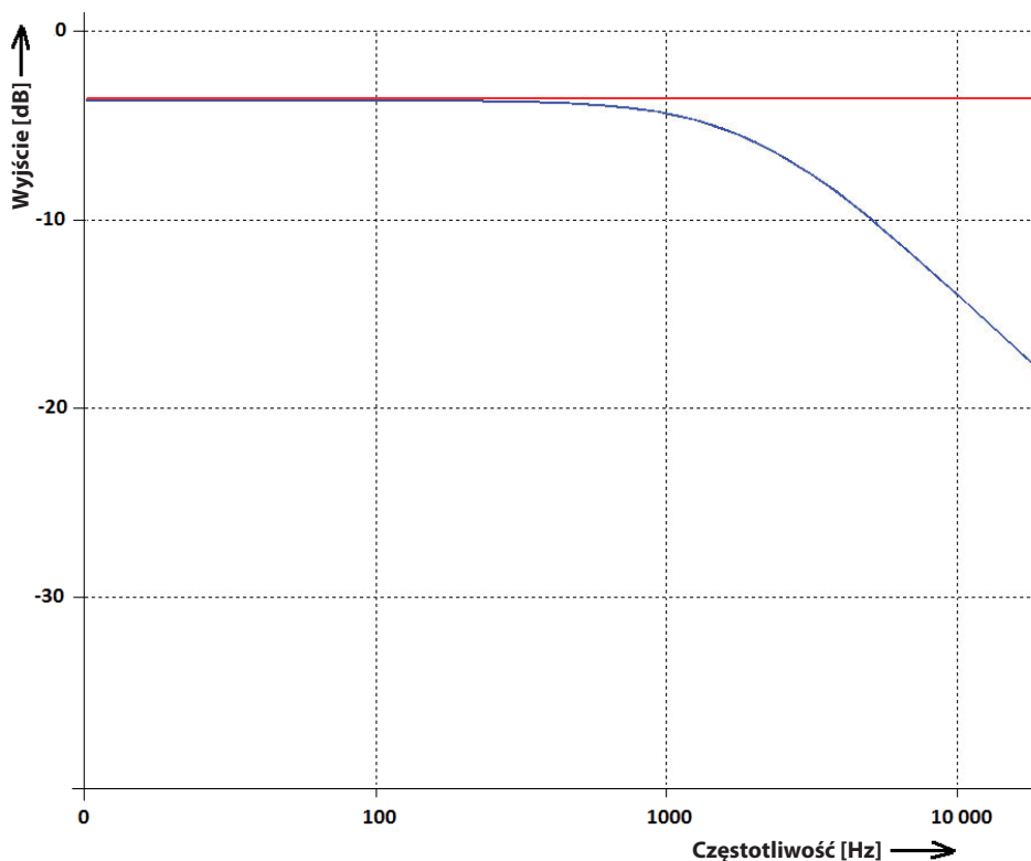
Odpowiedź częstotliwościowa źródeł dźwięku: wielopunktowego jedno osiowego (niebieska) i punktowego (czerwona)
